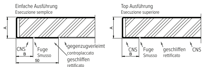
Schnitt A-A / Intaglio A-A
