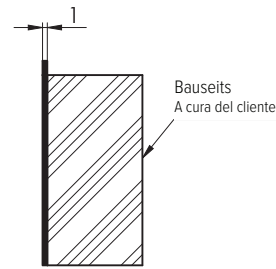
Schnitt A-A / Intaglio A-A
