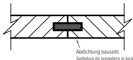
Detail Z / Dettaglio a Z
