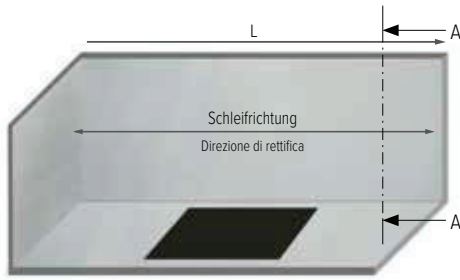
Schnitt A-A / Intaglio A-A
