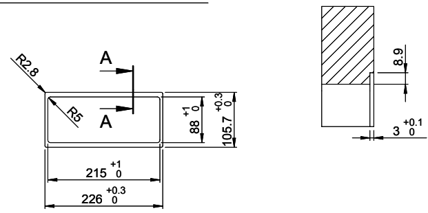
A-A (1 : 2)
