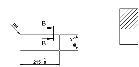
B-B (1 : 2)
