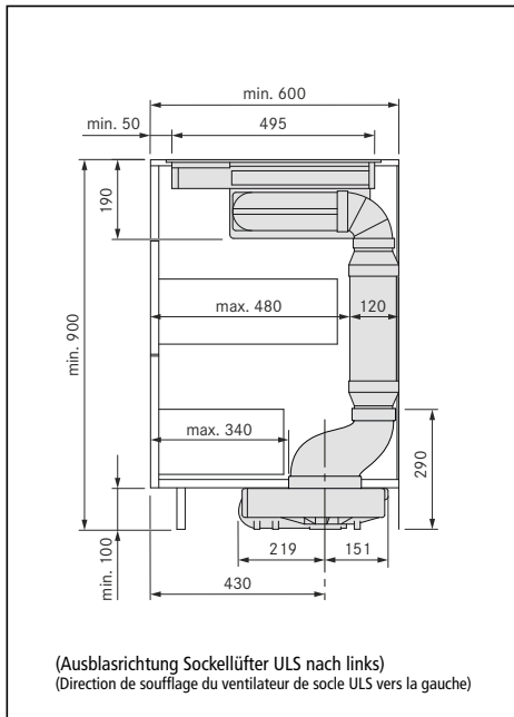
Einbauschchnitt CKA2 mit Flachschalldämpfer USDF (600 mm) Coupe de montage CKA2 avec silencieux plat USDF (600 mm)
