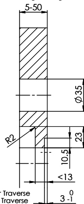
A-A (1 : 2)
