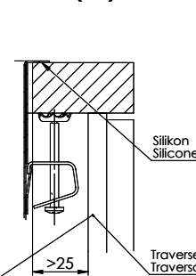
Z (1:2)
