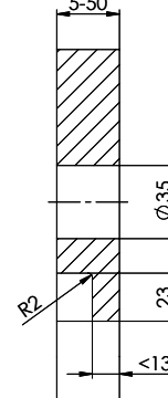
B-B (1 : 2)
