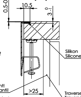
Z (1:2)
