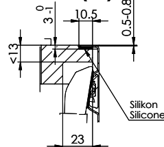
Y (1:2)
