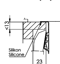
Y (1:2)
