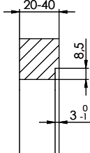
A-A (1 : 2)
