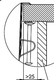
DETAIL Y MABSTAB 1 : 2
