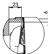
DETAIL x MABSTAB 1:2
