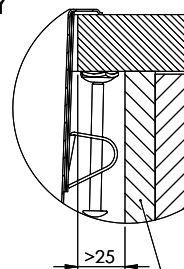
DETAIL Y MAßSTAB 1:2
