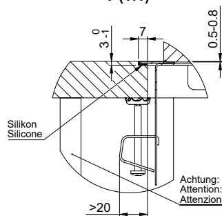
Y (1:1)
